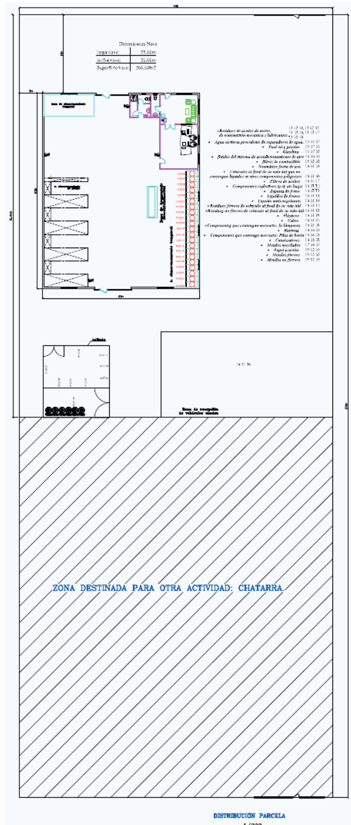
Figura 1. Plano en planta de la parcela.
