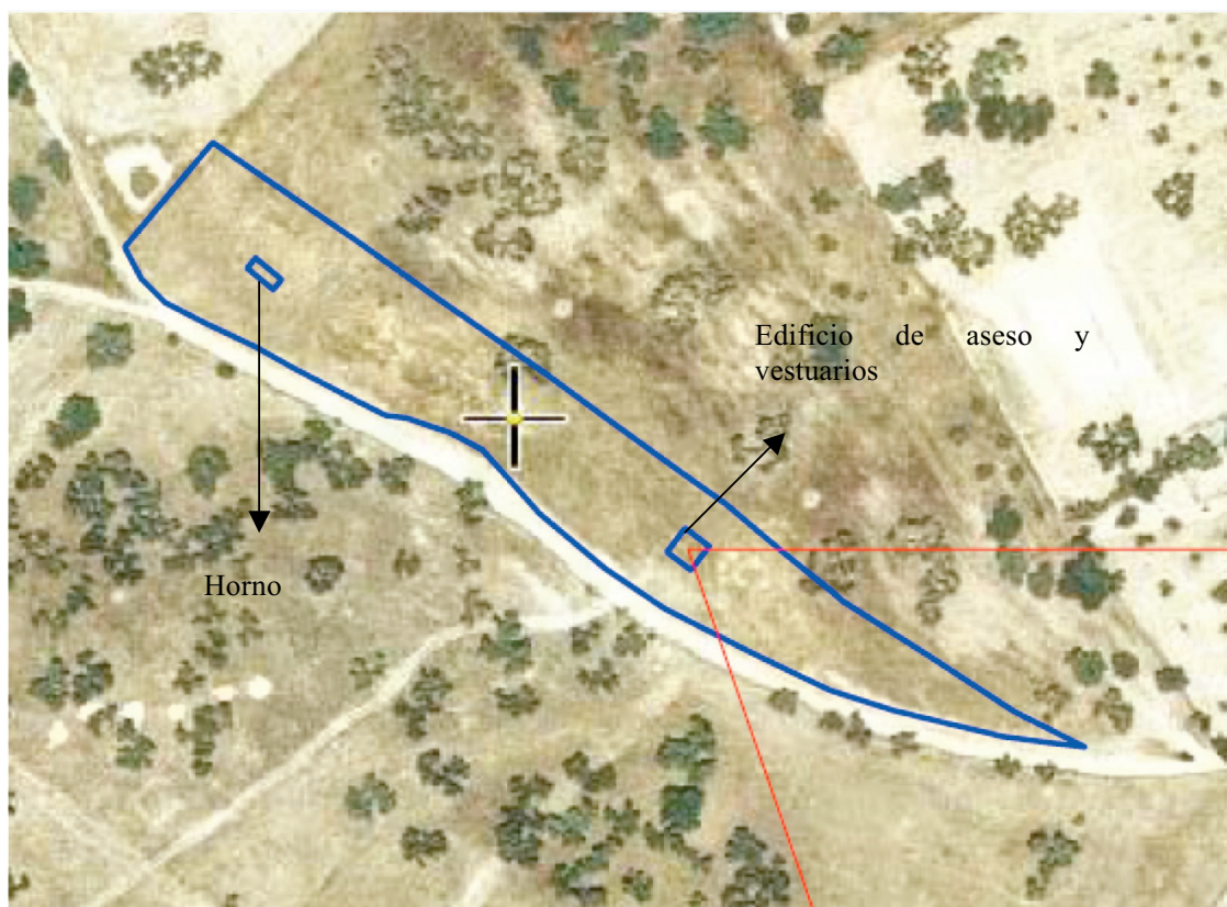
Figura 1 Plano en planta de la instalación.
