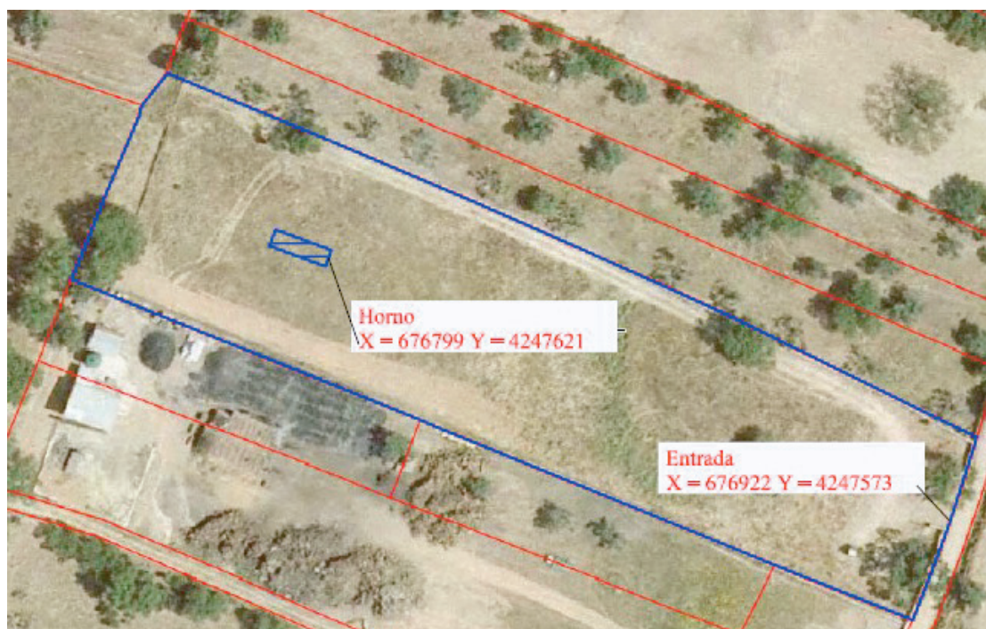
Figura 1 Plano en planta de la instalación.
