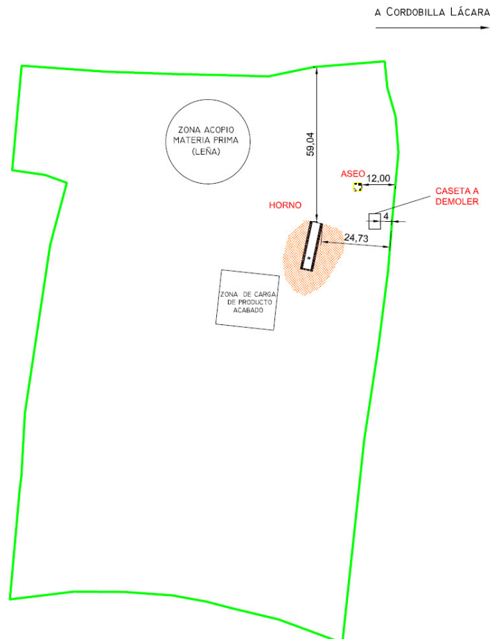
Figura 1 Plano en planta
