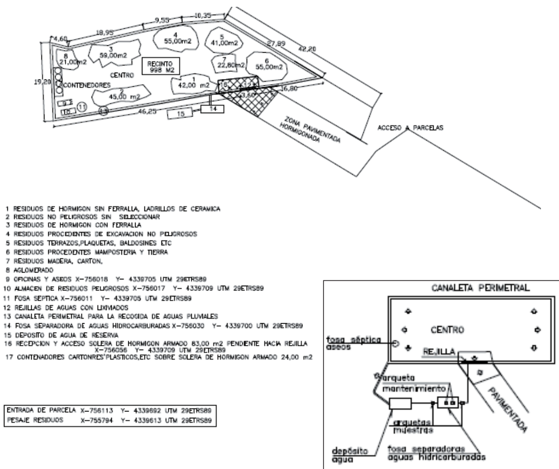
Figura 1. Plano en planta de las instalaciones
