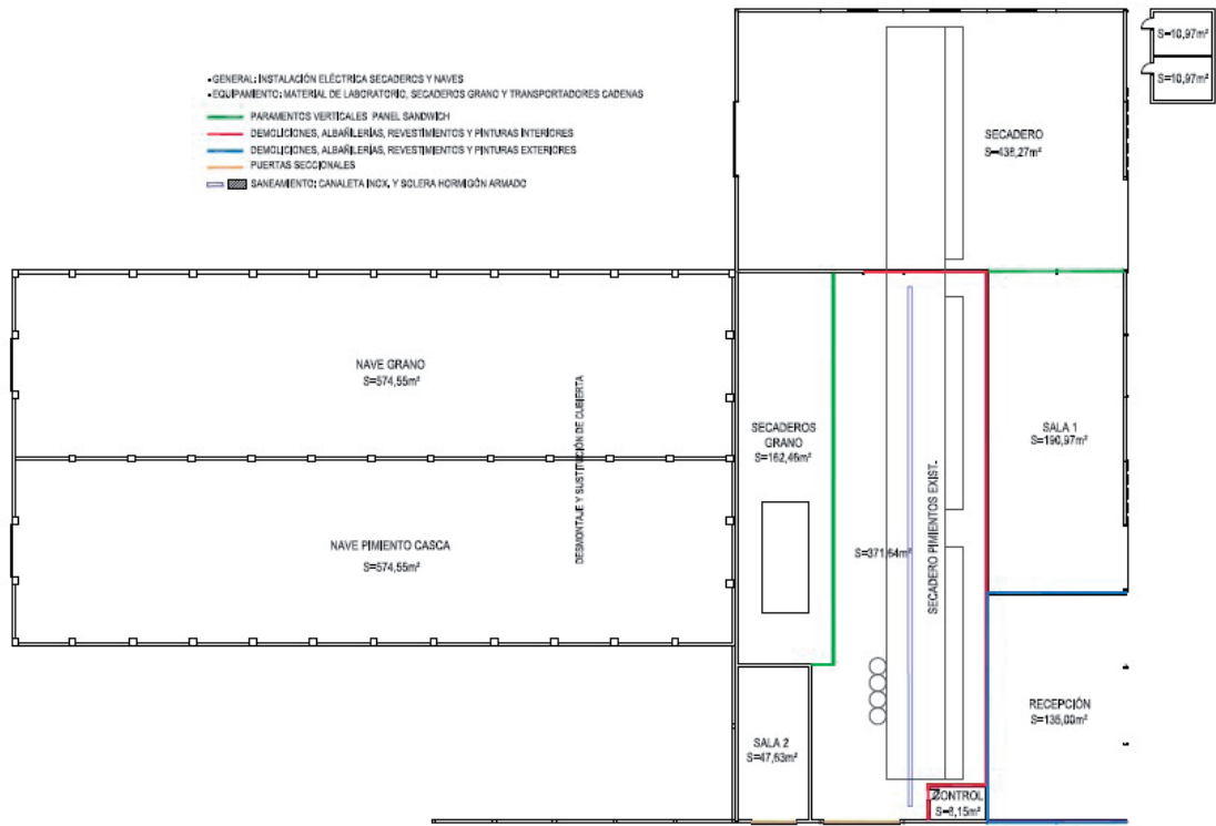
Fig. 1. Planta general de la industria.
