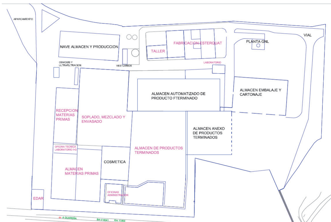
Figura 1. Plano de distribución de las instalaciones y edificaciones principales.
