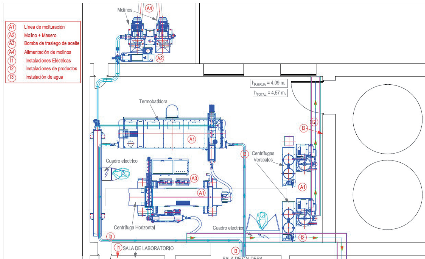
Fig. 1. Situación proyectada de las instalaciones
