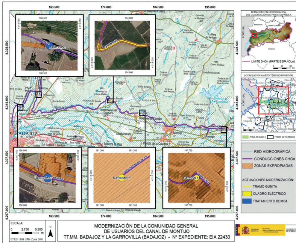
Plano de situación de las actuaciones proyectadas. (Fuente: CHG).
