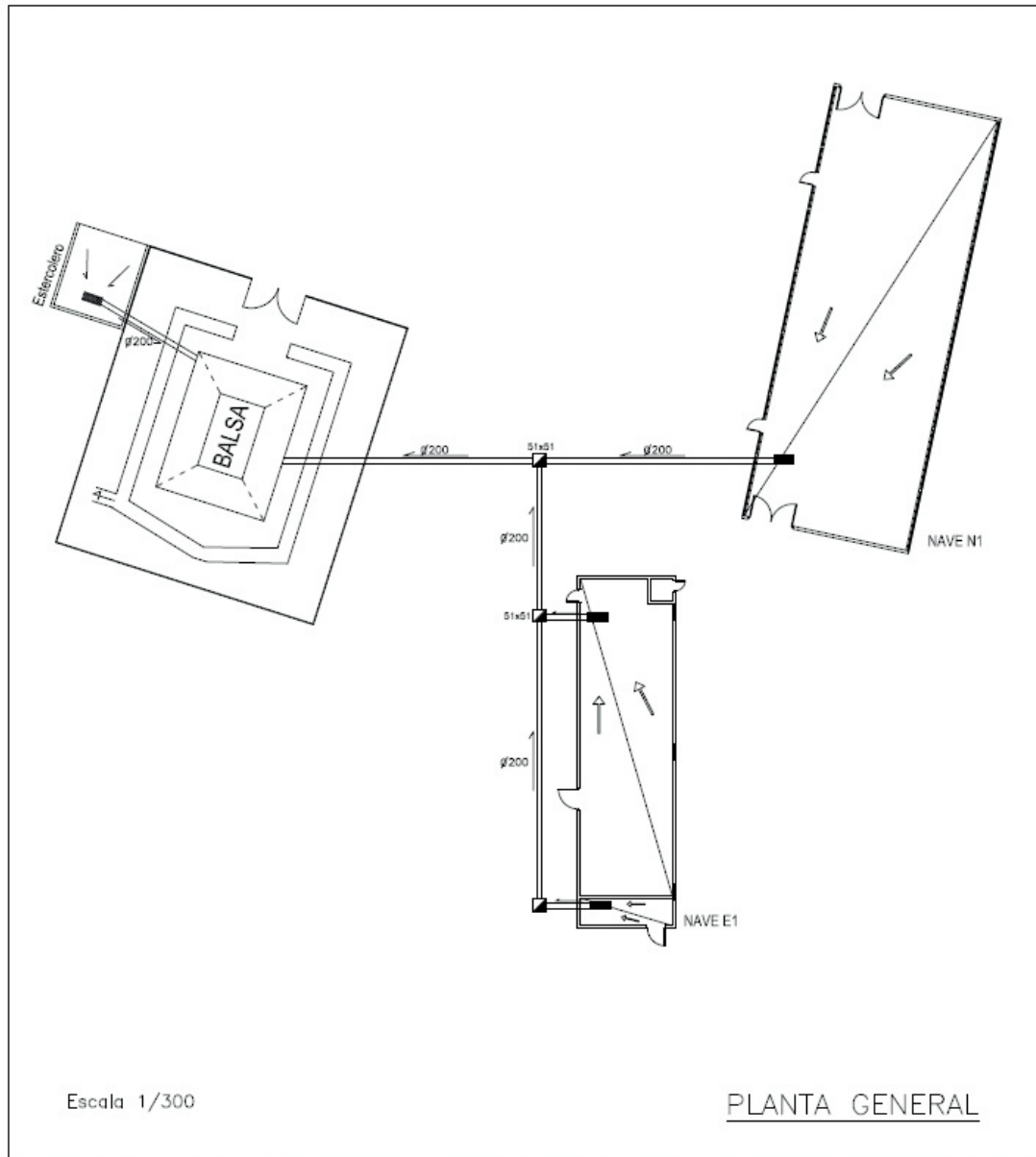
Fig. 1. Planta general de las instalaciones.
