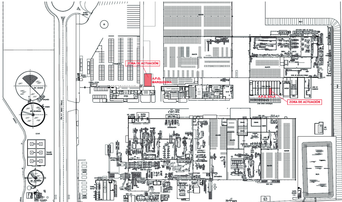
Plano n.º 1. Ubicación marquesina almacenamiento productos químicos
