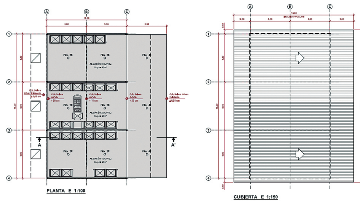
Plano n.º 1. Ubicación marquesina almacenamiento productos químicos
