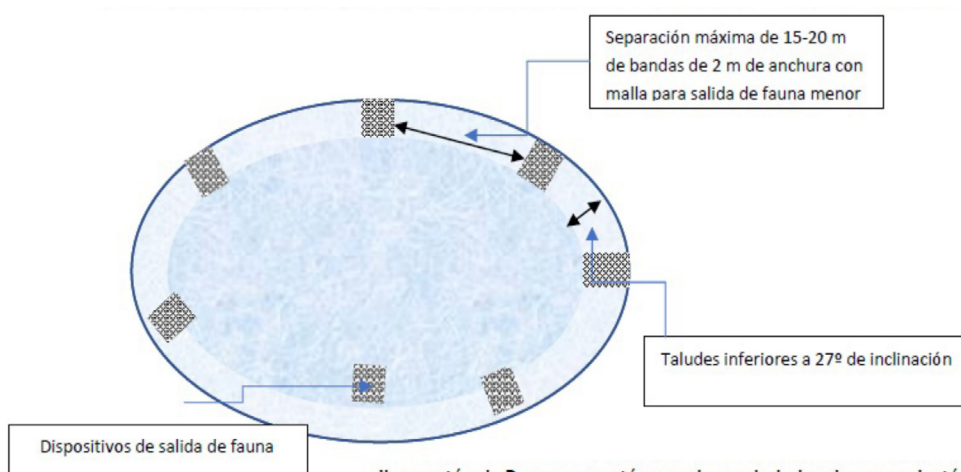
Ilustración I: Representación en planta de balsa de acumulación y dispositivos de salida de fauna menor
