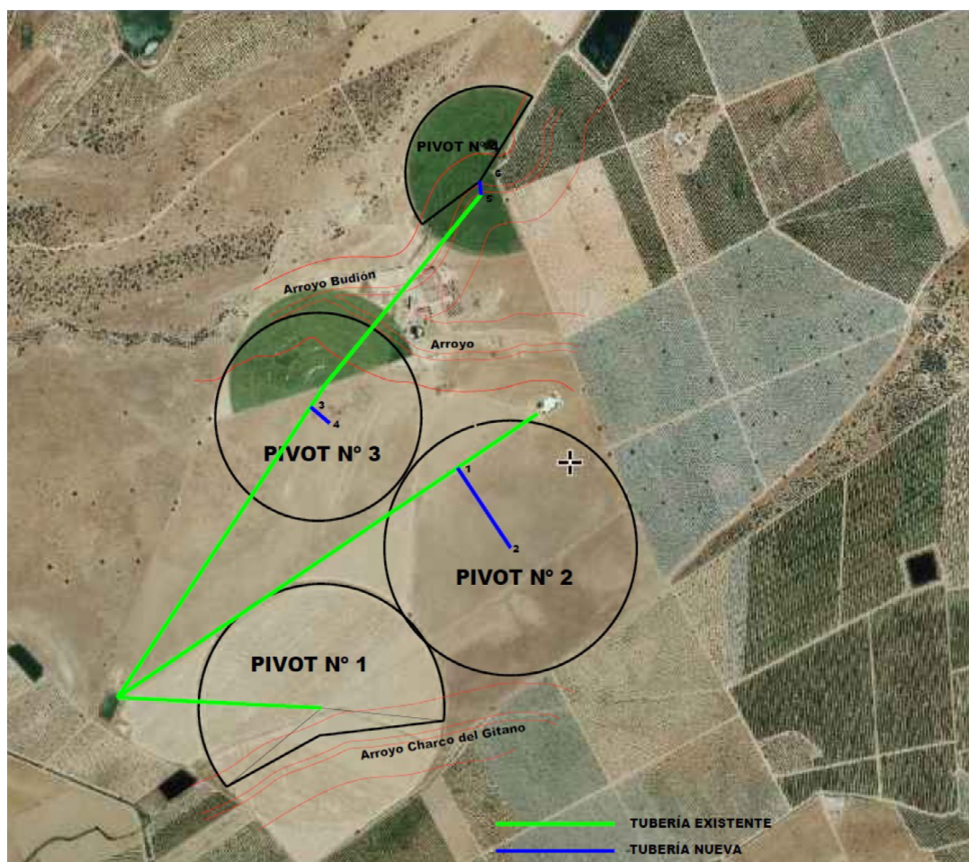
Plano 3. Red de riego y Pivots (Fuente: Estudio de Impacto Ambiental).
