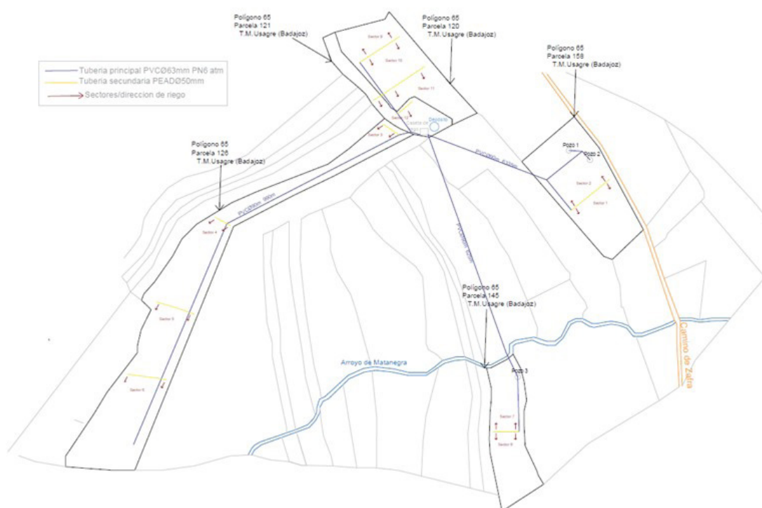
Plano 2: Distribución de las instalaciones de riego (Fuente: Documento Ambiental)
