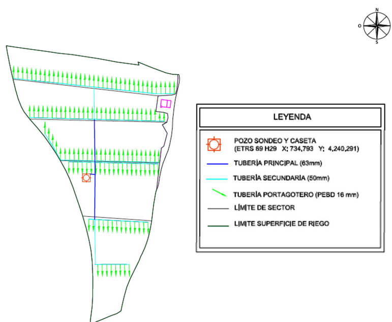
Plano 2: Distribución de las instalaciones de riego (Fuente: Documento Ambiental)
