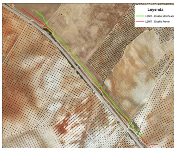
Comparativa de modificación de la línea de evacuación. Fuente: Documento Ambiental
