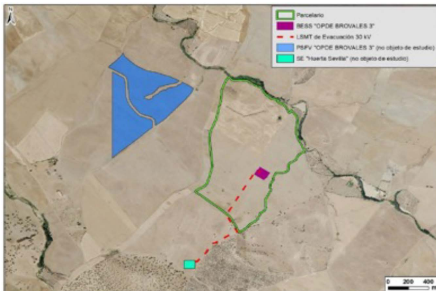
Proyecto de hibridación BESS OPDE Brocales 3. Fuente: documento ambiental
