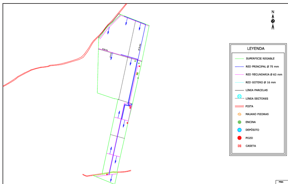
Plano de distribución del riego. (Fuente: Documento ambiental).
